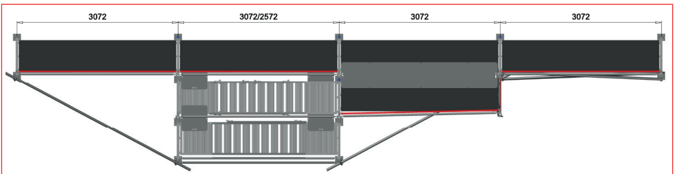
Fig. 3.10: Utv trapp dobbelt løp sett ovenfra
