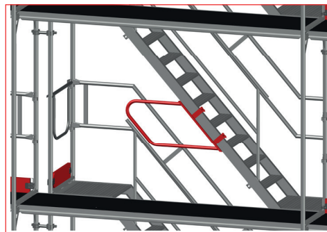
Fig. 3.4: Rekkverk underside trapp
