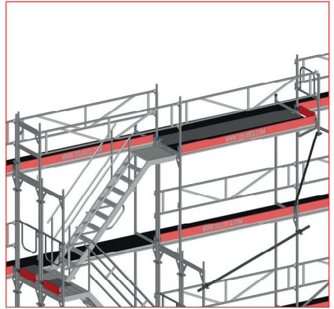
Fig. 3.7: Utv trapp dobbelt løp detail B
