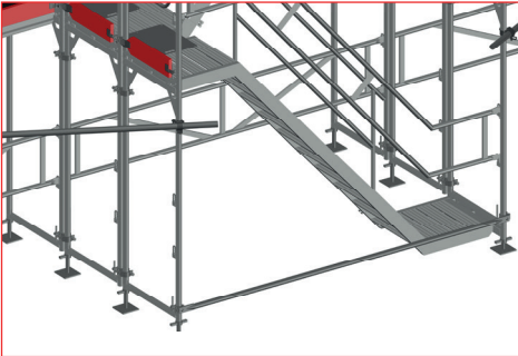
Fig. 3.8: Utv trapp dobbelt løp detail A
